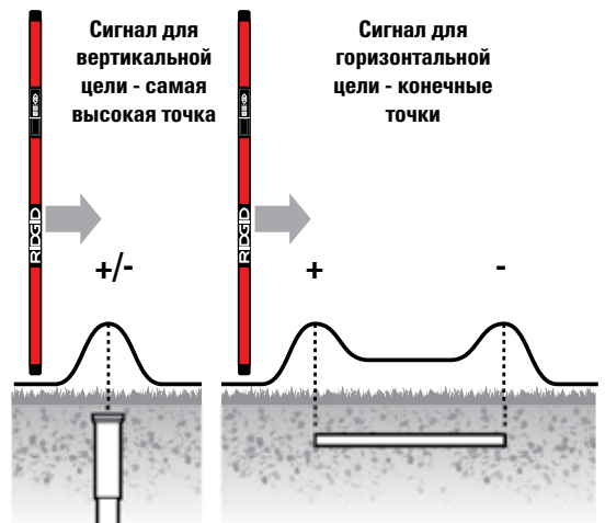
Сигналы и полярность вертикальных и горизонтальных целей
